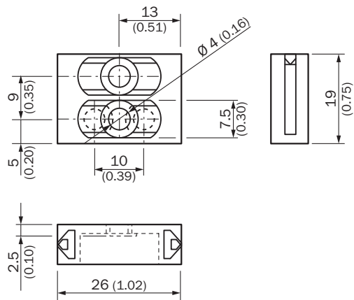
Габаритный чертеж: BEF-SLG2
