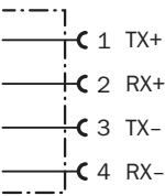
Схема соединений RS-485
