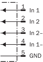
Схема соединений энкодера
