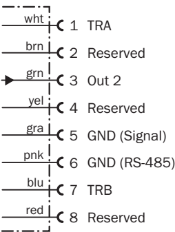
Схема соединений энкодера
