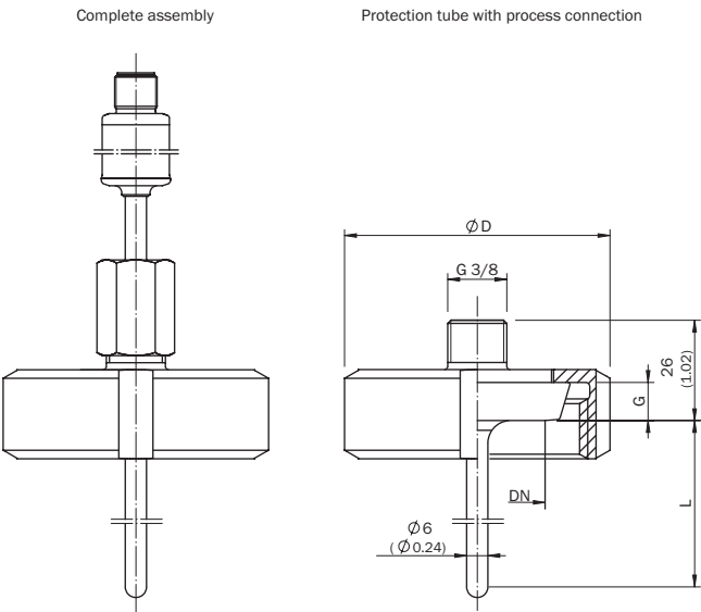
Габаритный чертеж
